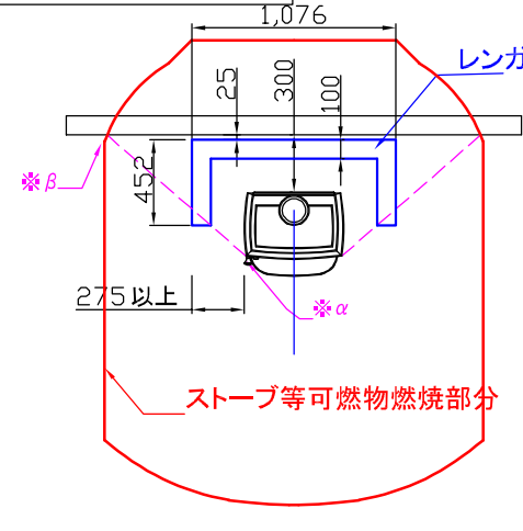
平面図 平行設置 レンガ積み
