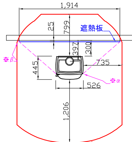
平面図 平行設置 ストーブ等可燃物燃焼部分
