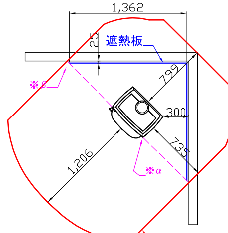
平面図 コーナー設置 ストーブ等可燃物燃焼部分
